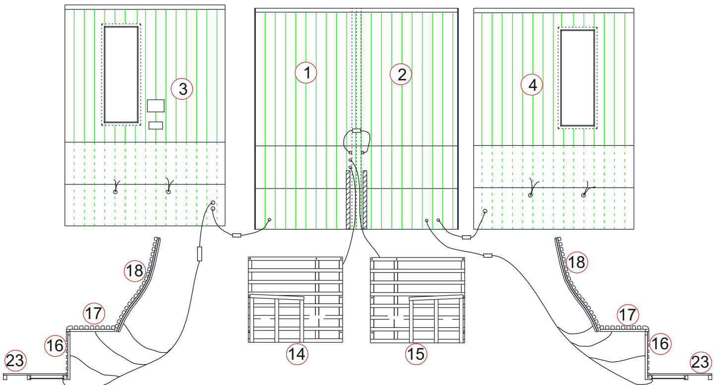
Anschlussplan
